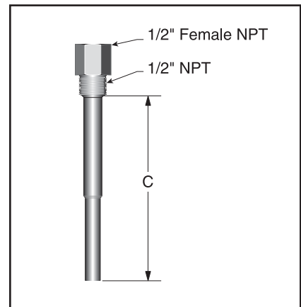
Thermowell
